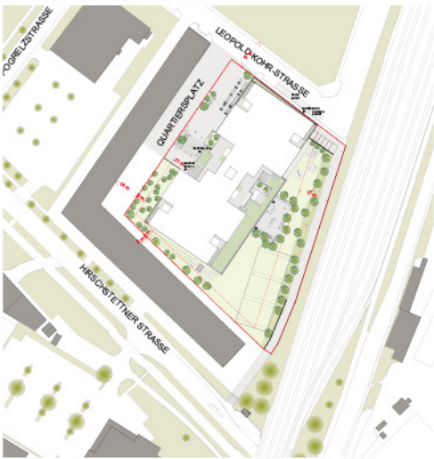
LAGEPLAN 1:500
