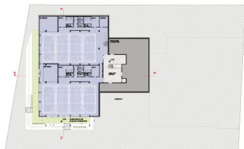
GRUNDRISS UNTERGESCHOBIS 1:200
