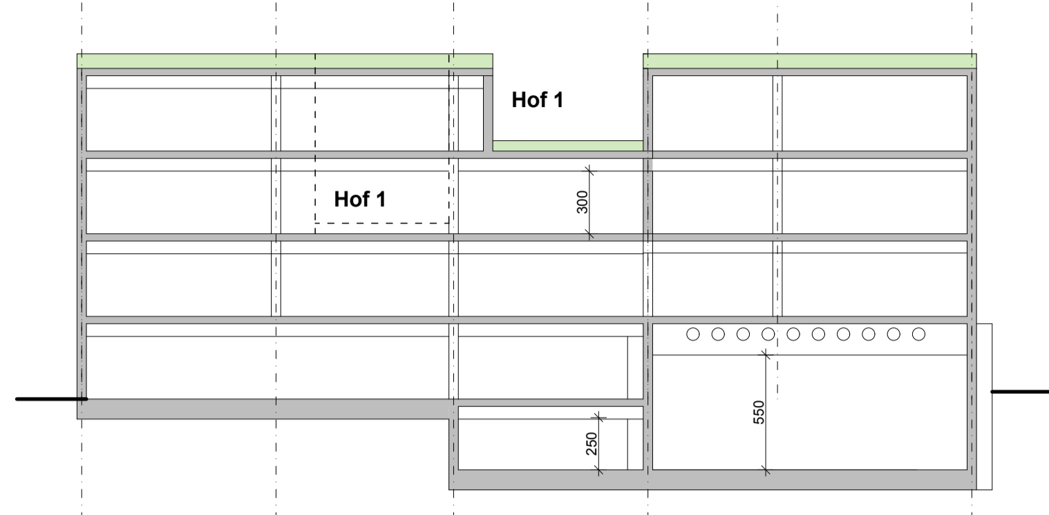
Schnitt Turnhalle
