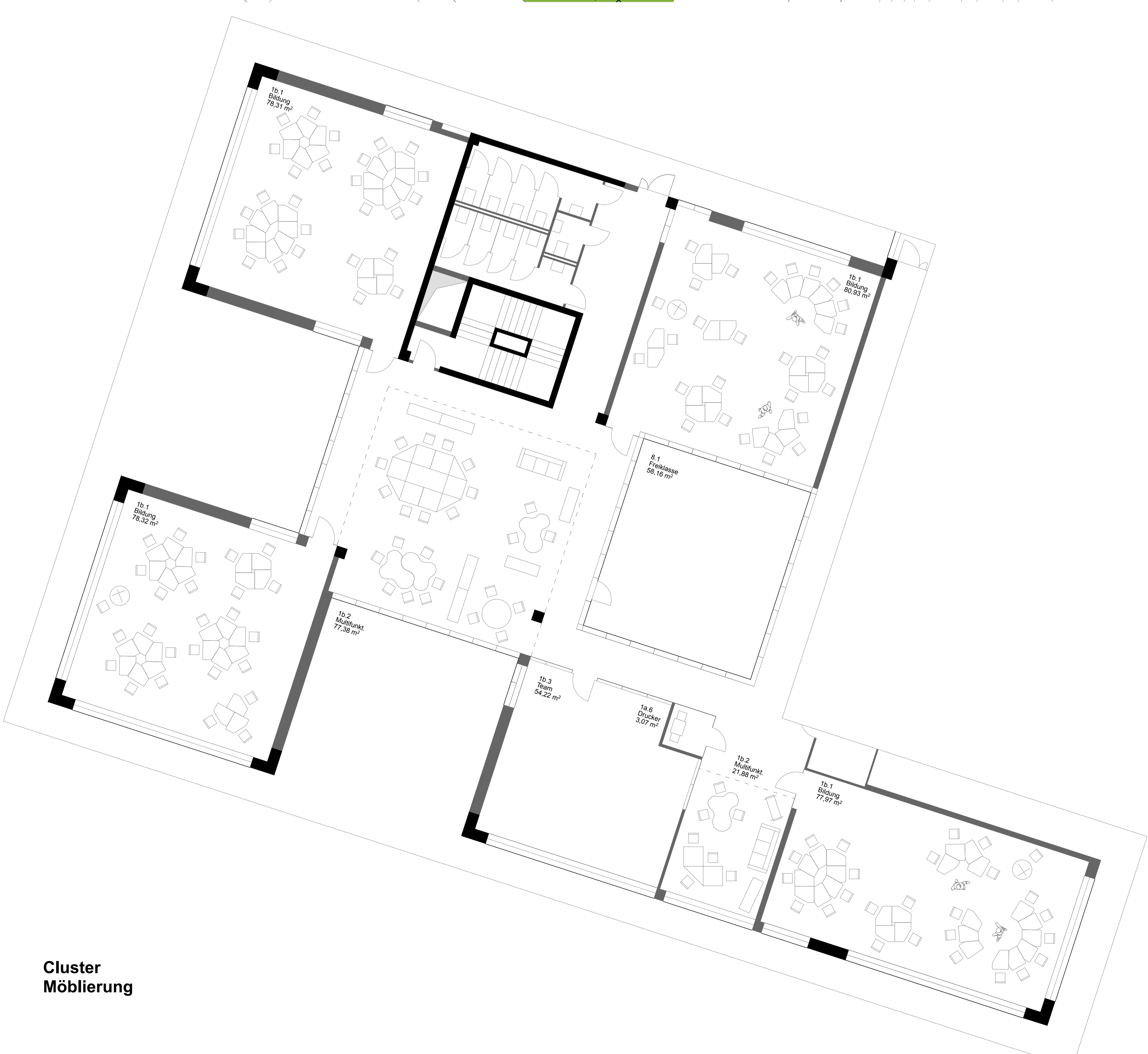
Erdgeschoß
