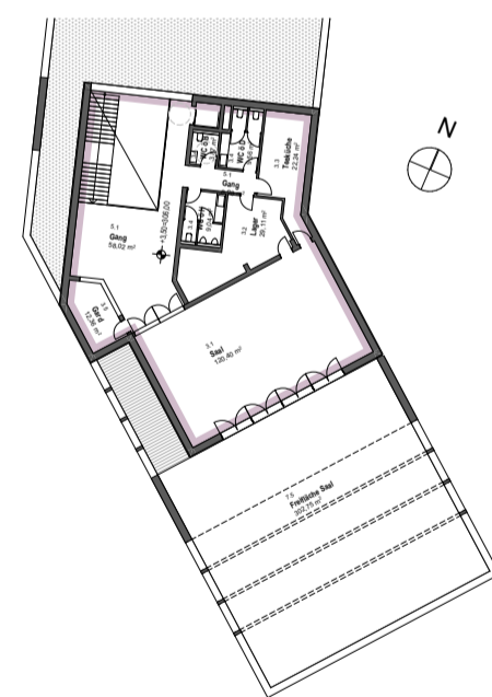
OBERGESCHOSS 1:200
