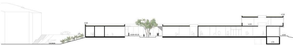
LÄNGSSCHNITT C-C M.1:200
